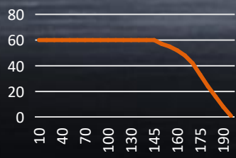
48V T-N曲线 (T-N under 48V)
